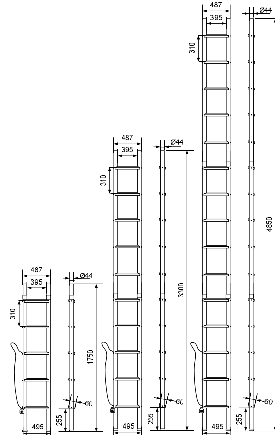
Рис. 1. Габаритные размеры (одно звено)
